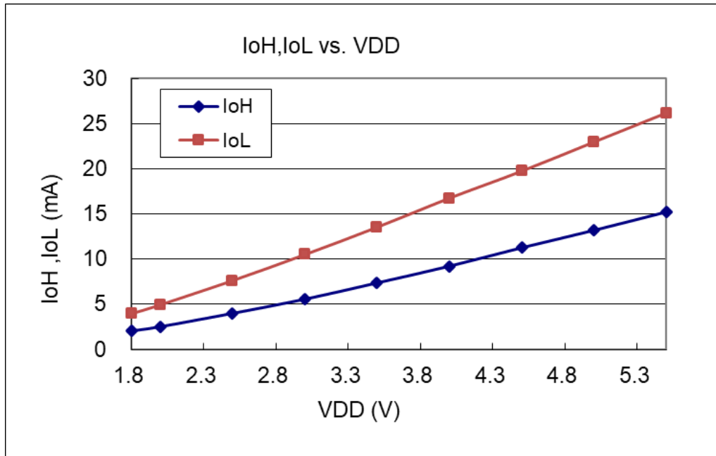
4.13. 引脚输出驱电流( I_{OH} )与灌电流( I_{OL} ) 曲线图
