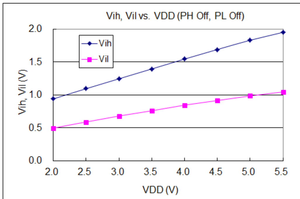
4.14. 引脚输出输入高电压与低电压( V_{IH} / V_{IL} ) 曲线图
